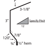
18 Jamb Trim PF21
